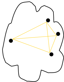
cohesion
